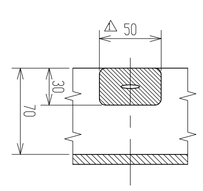
断面 A-A S=1:2 (16ヶ所)
