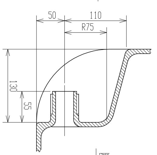
断面 A-A S=1:2 (16ヶ所)
